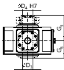
P4DV 带锁紧盘的空心轴
