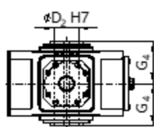
V3HV 空心轴
