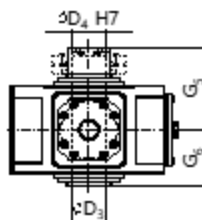
V3DV 带锁紧盘的空心轴
