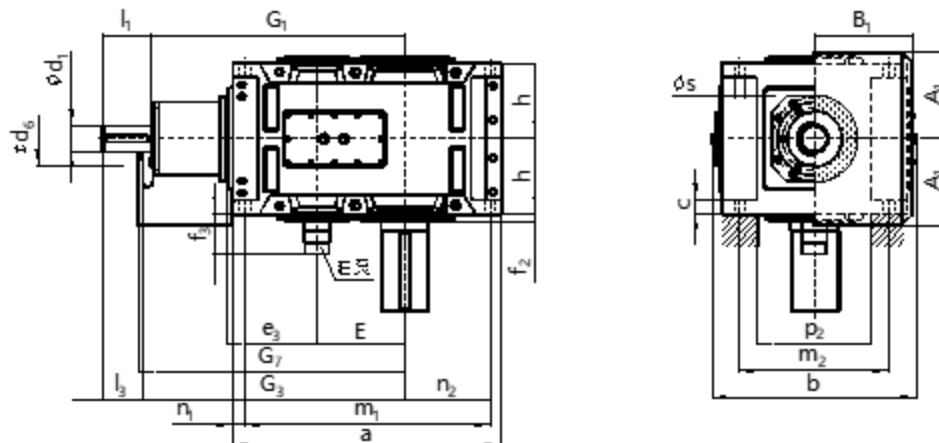
V2HV 空心轴
