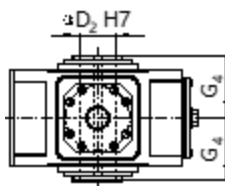
V2HV 空心轴
